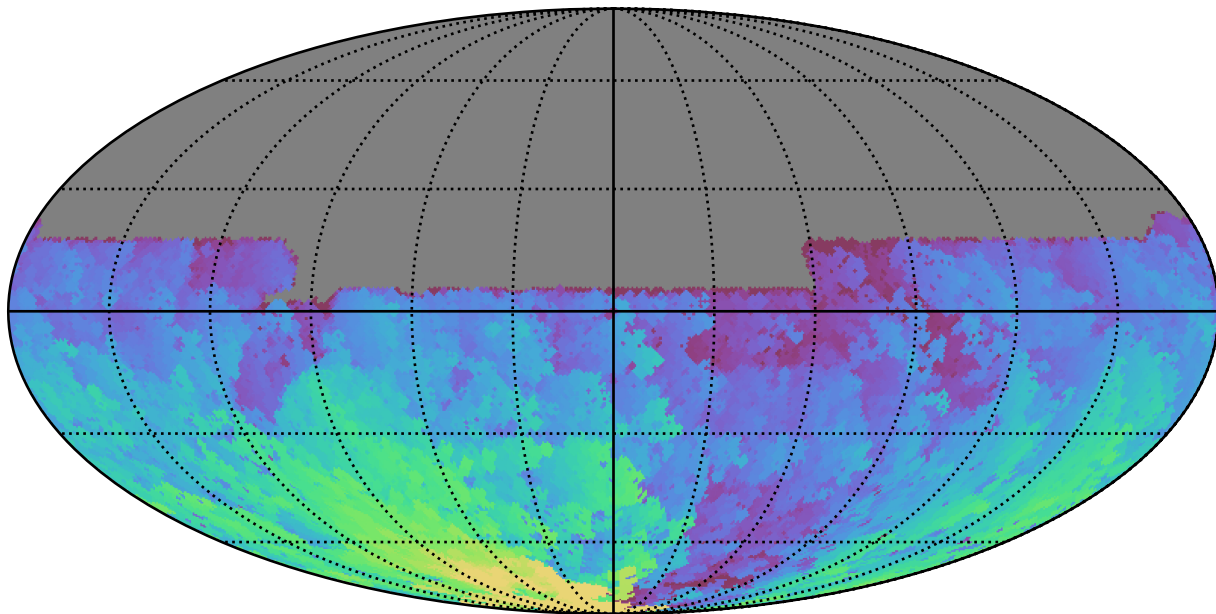
weather_cloudso14v3.4_10yrs All sky u band: Max HA
