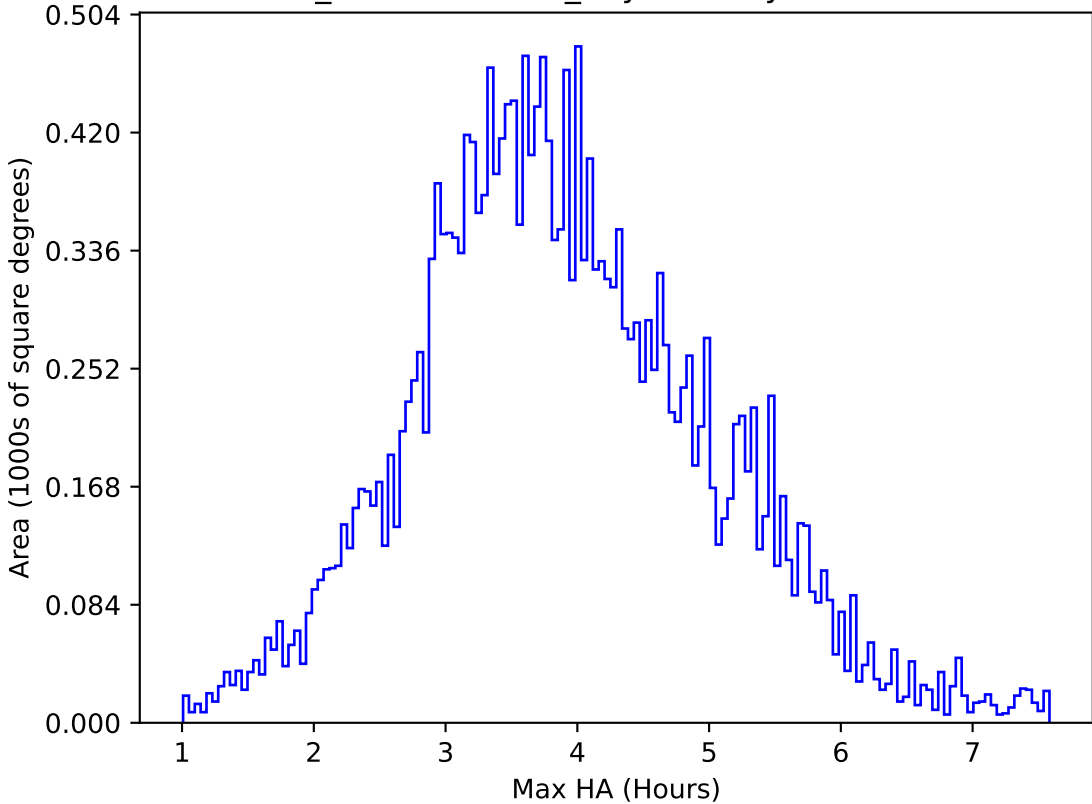
weather_cloudso14v3.4_10yrs All sky u band: Max HA
