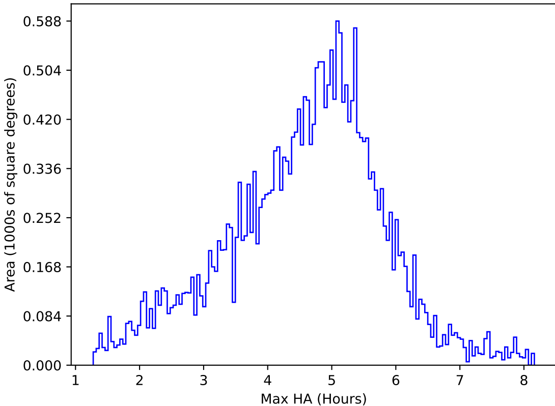
weather_cloudso14v3.4_10yrs All sky i band: Max HA
