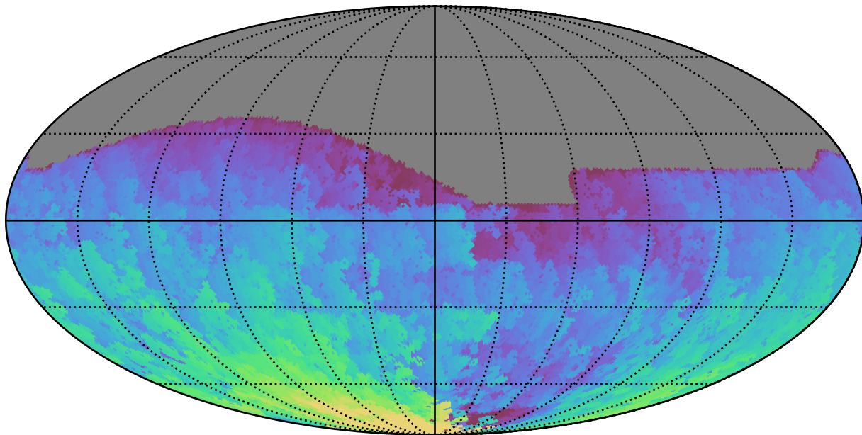
weather_cloudso14v3.4_10yrs All sky g band: Max HA
