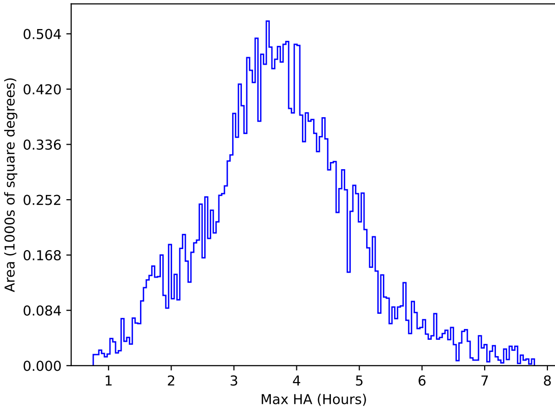
weather_cloudso14v3.4_10yrs All sky g band: Max HA
