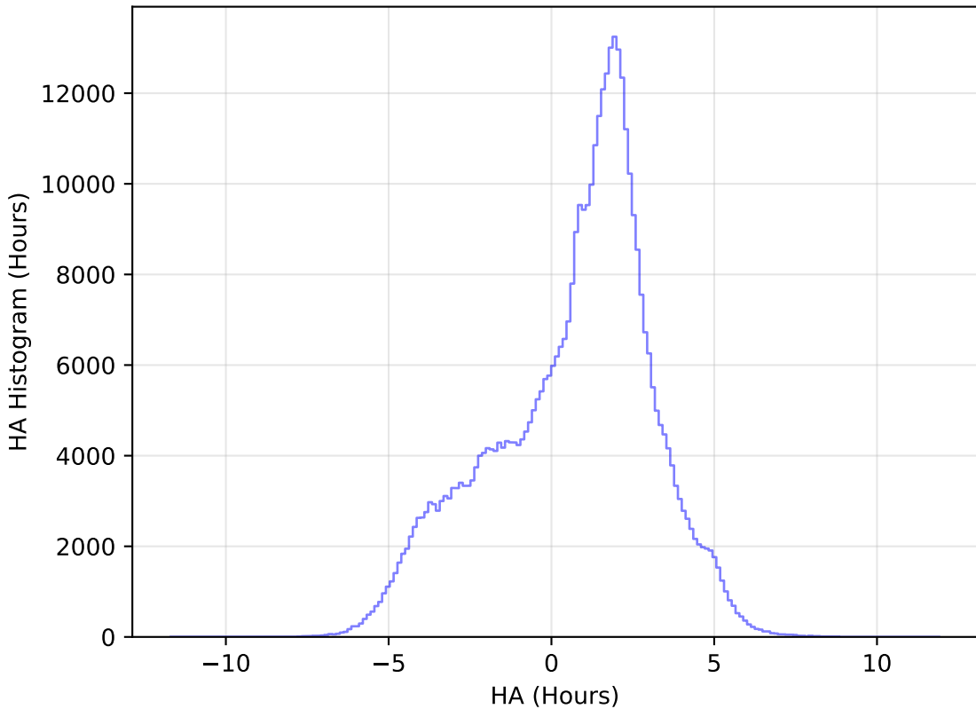
weather_cloudso14v3.4_10yrs WFD z band: HA Histogram
