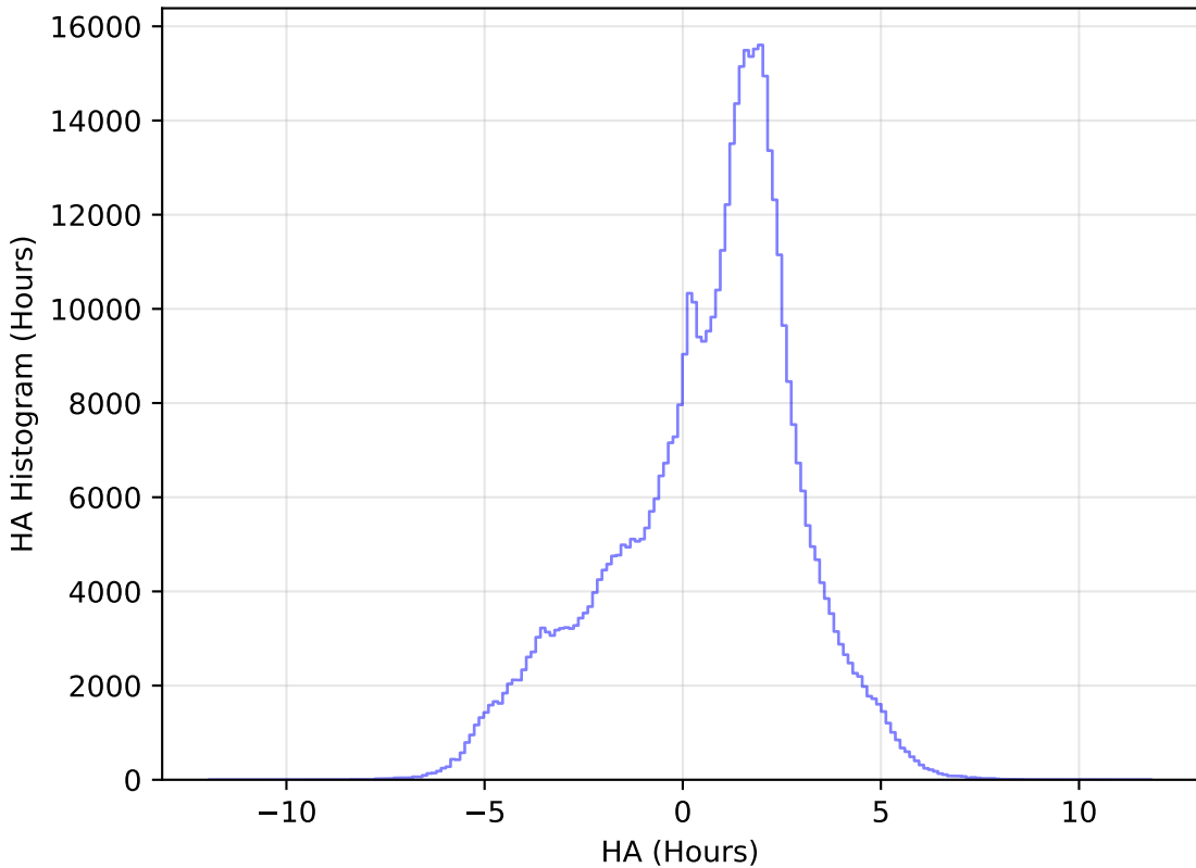
weather_cloudso14v3.4_10yrs WFD i band: HA Histogram
