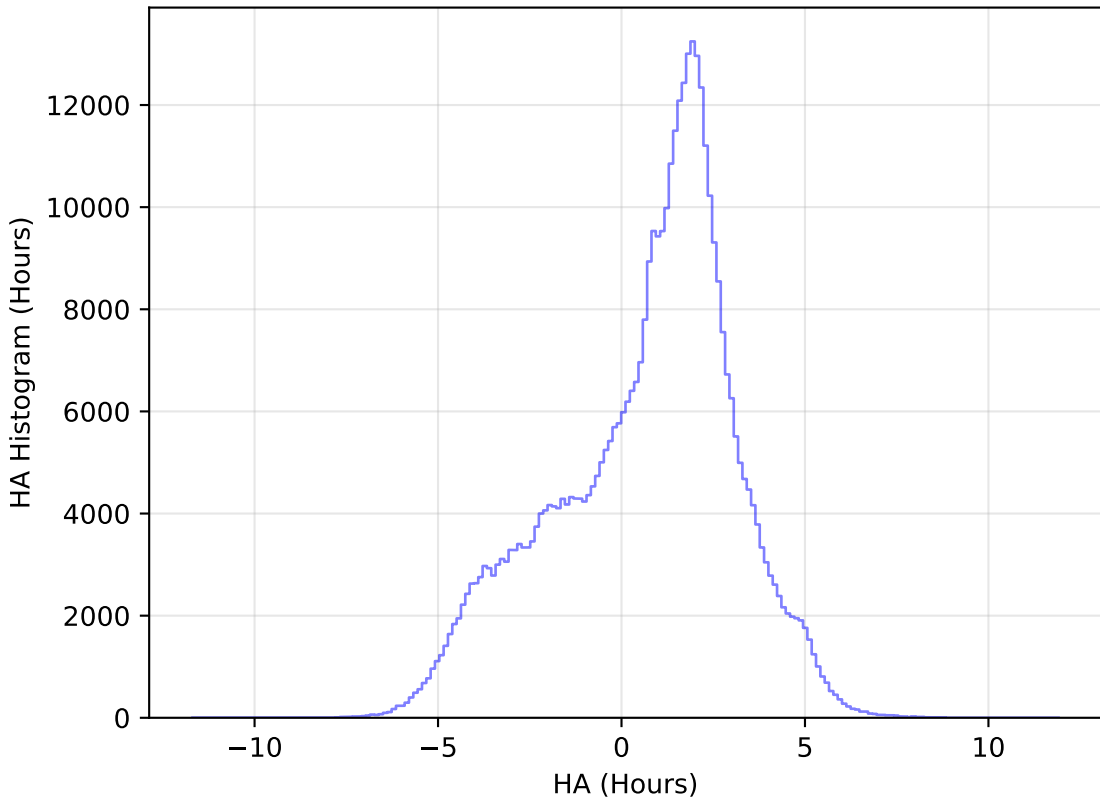
weather_cloudso14v3.4_10yrs All sky z band: HA Histogram
