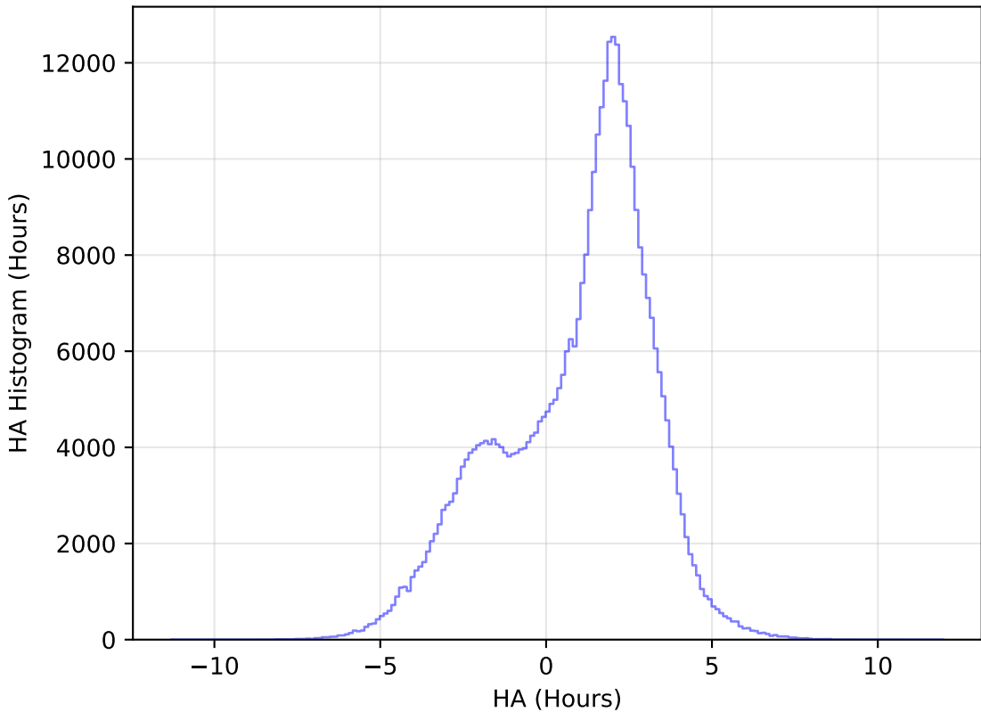
weather_cloudso14v3.4_10yrs All sky y band: HA Histogram
