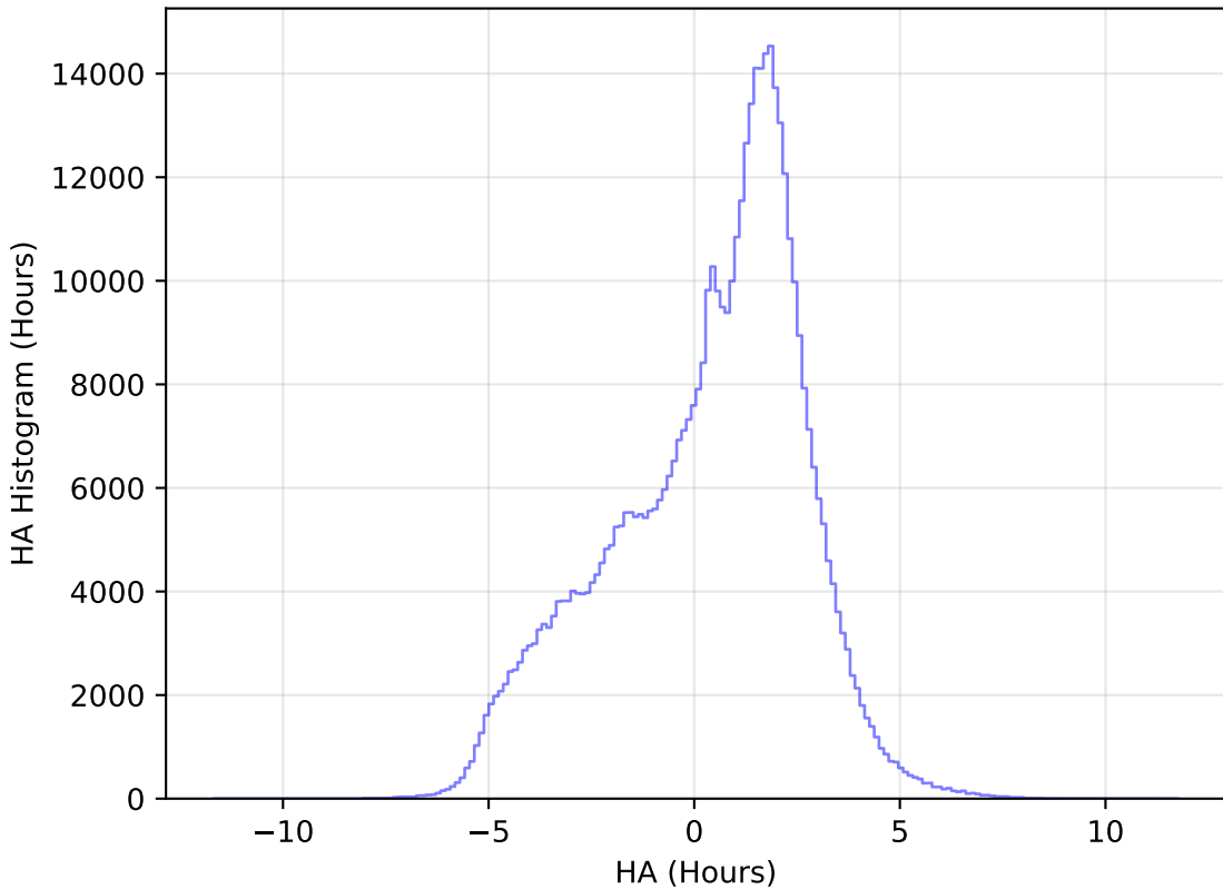
weather_cloudso14v3.4_10yrs All sky r band: HA Histogram
