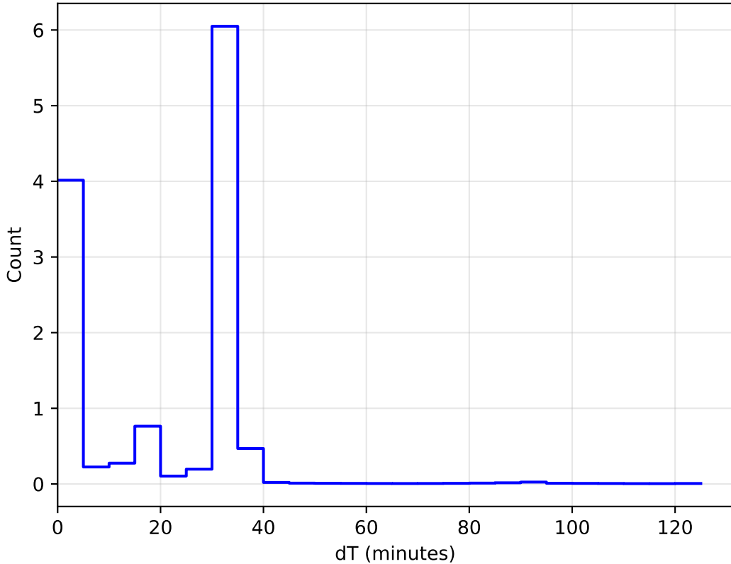
weather_cloudso14v3.4_10yrs WFD: DeltaT Histogram
