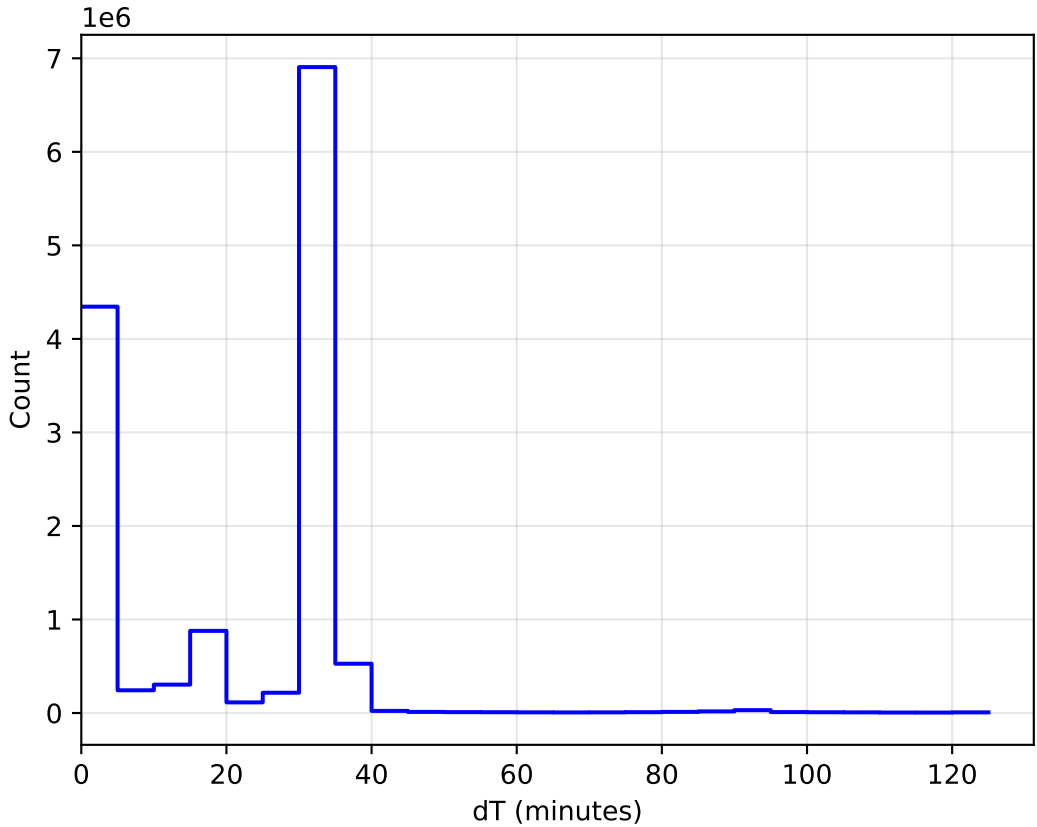
weather_cloudso14v3.4_10yrs All sky: DeltaT Histogram
