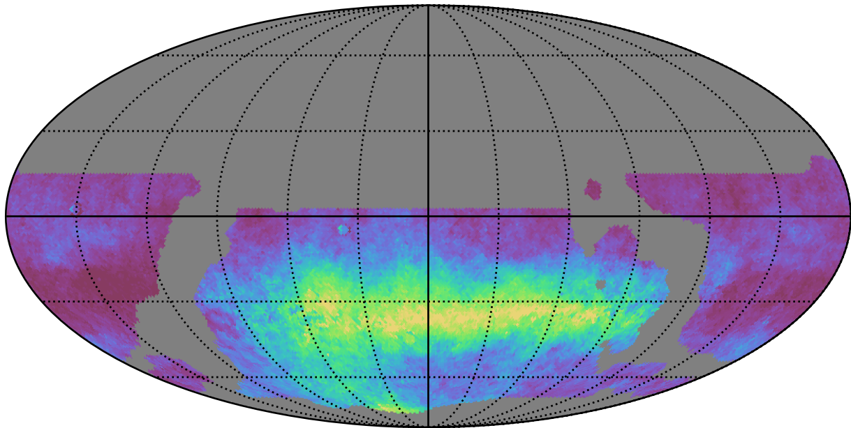
weather_cloudso14v3.4_10yrs WFD y band: AngleRms rotSkyPos
