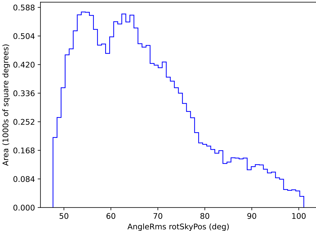
weather_cloudso14v3.4_10yrs WFD r band: AngleRms rotSkyPos
