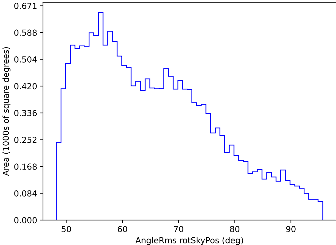
weather_cloudso14v3.4_10yrs WFD i band: AngleRms rotSkyPos
