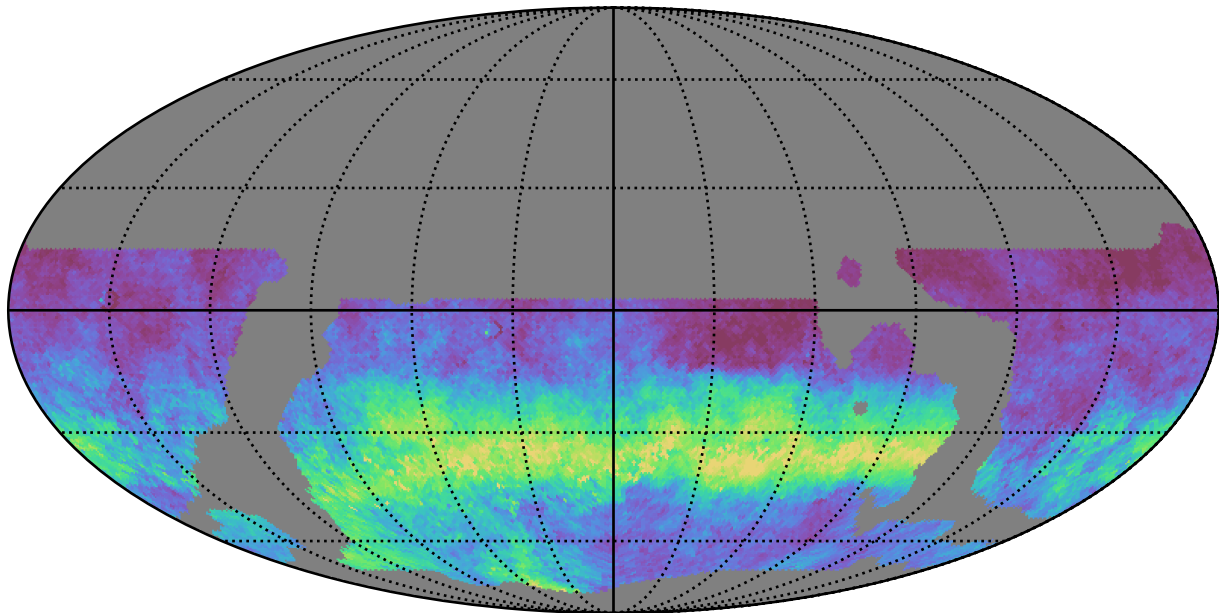
weather_cloudso14v3.4_10yrs WFD g band: AngleRms rotSkyPos
