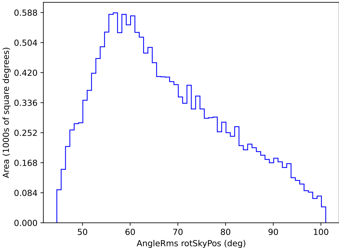
weather_cloudso14v3.4_10yrs WFD g band: AngleRms rotSkyPos
