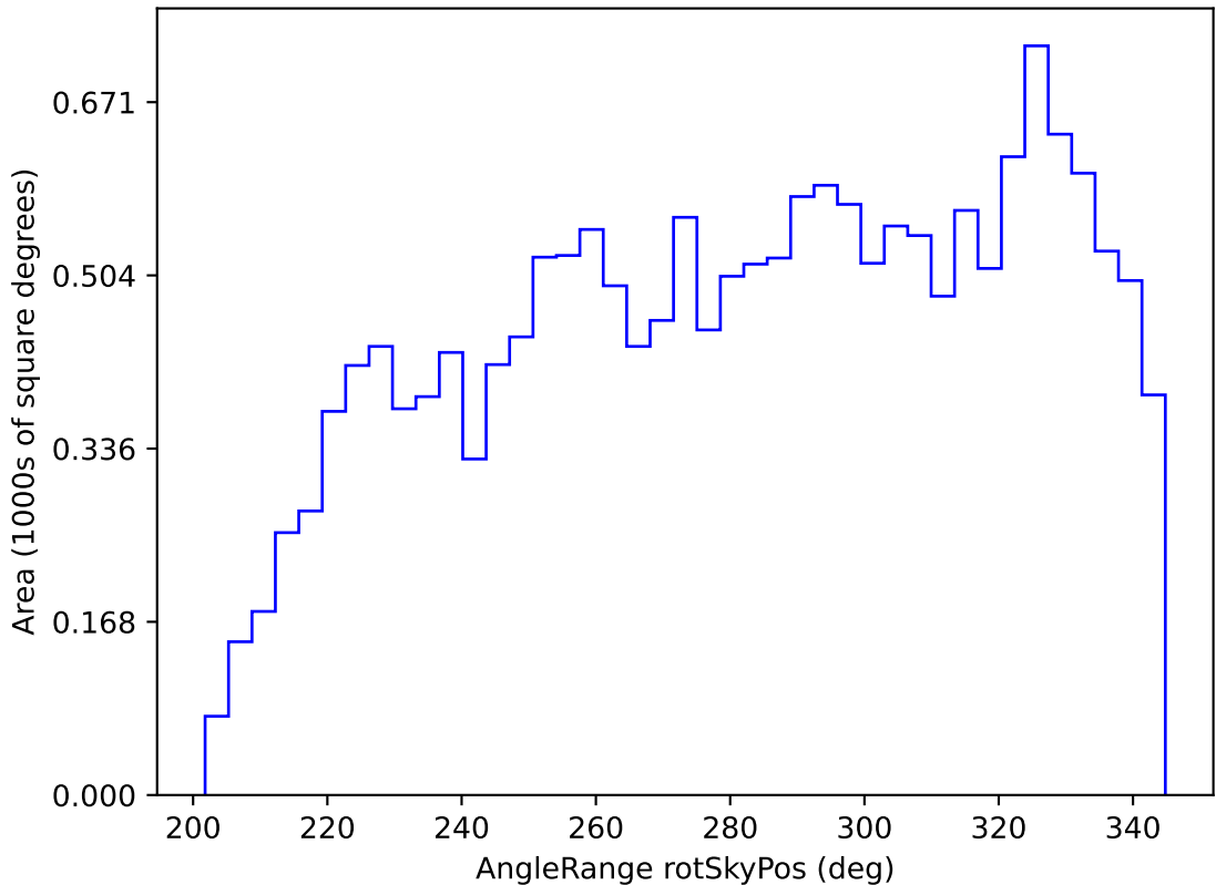
weather_cloudso14v3.4_10yrs WFD z band: AngleRange rotSkyPos
