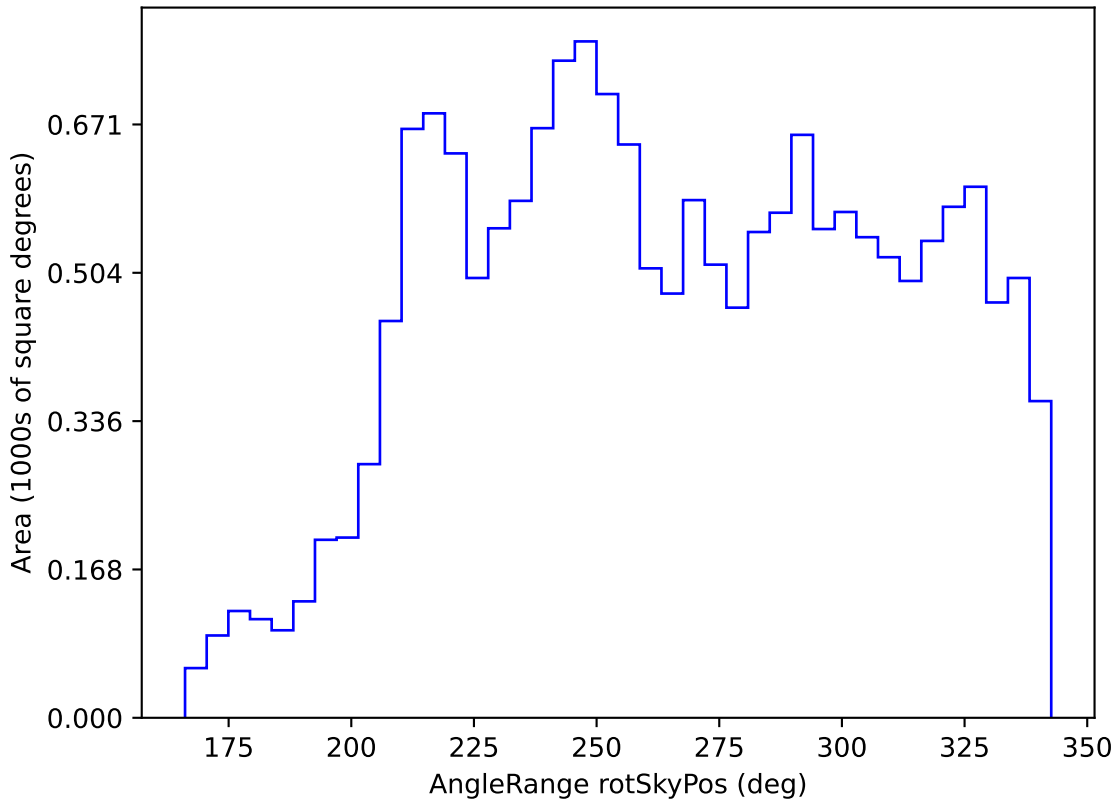
weather_cloudso14v3.4_10yrs WFD y band: AngleRange rotSkyPos
