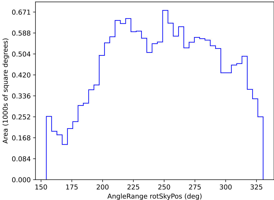
weather_cloudso14v3.4_10yrs WFD u band: AngleRange rotSkyPos
