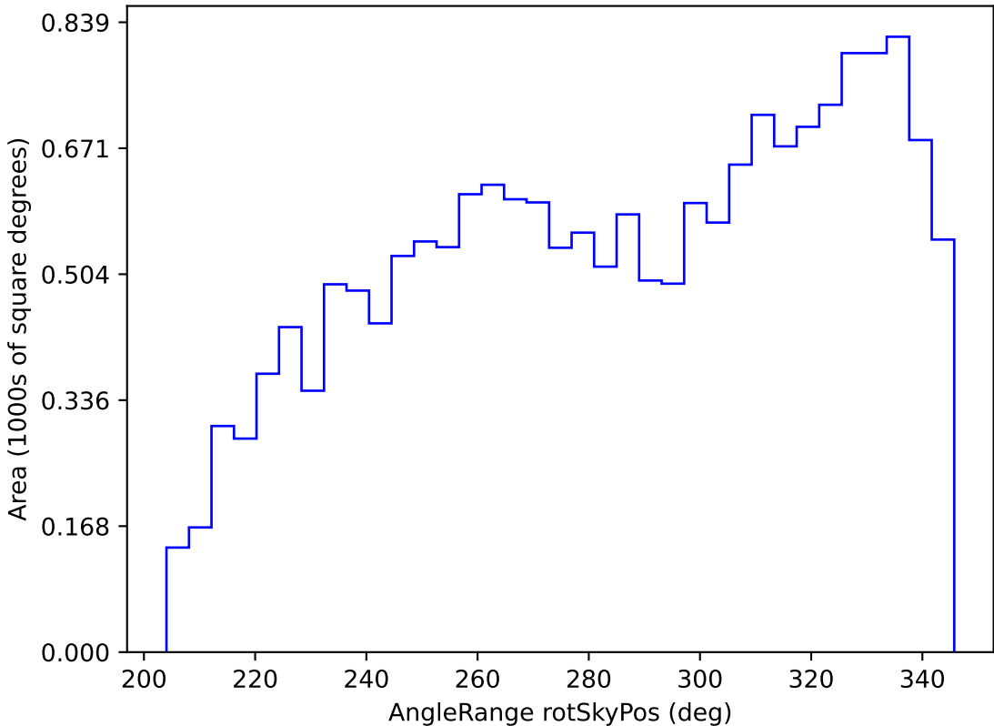
weather_cloudso14v3.4_10yrs WFD i band: AngleRange rotSkyPos
