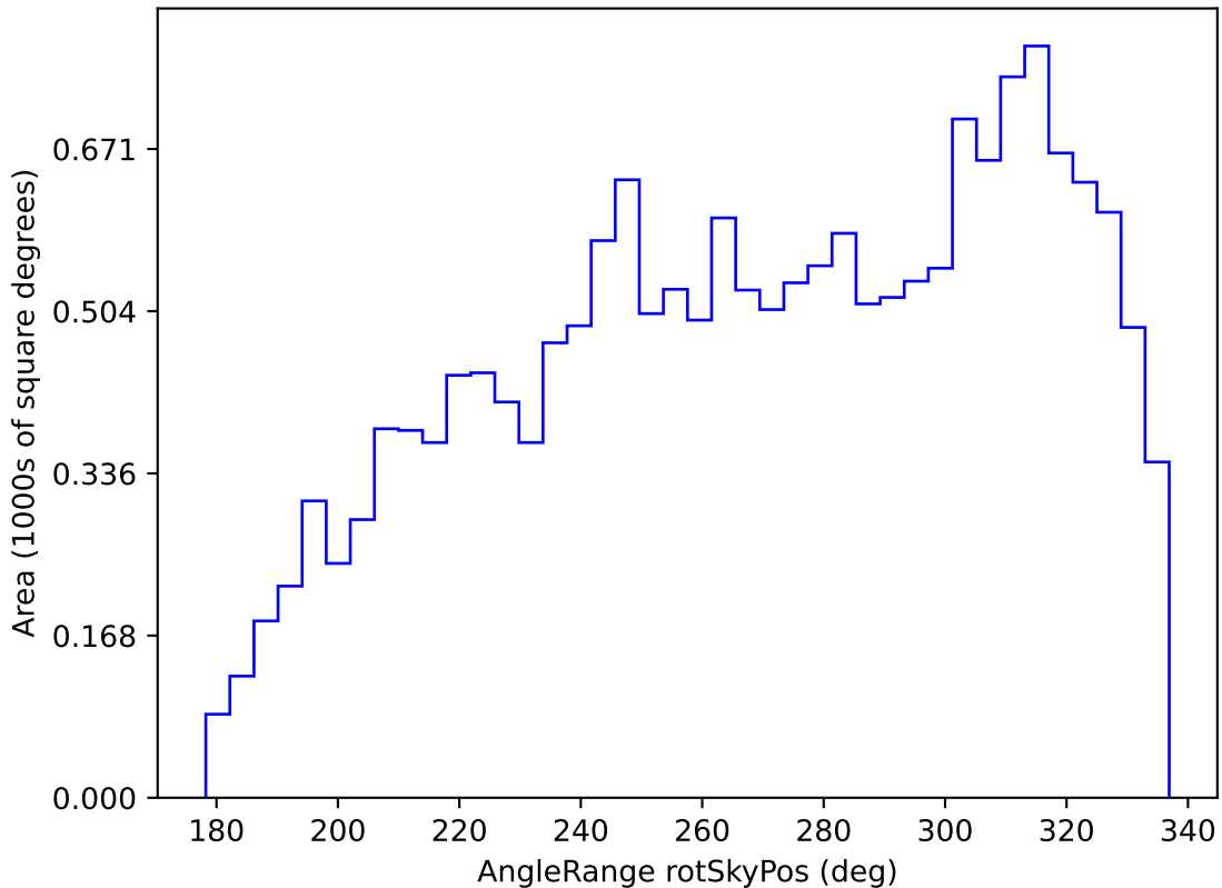
weather_cloudso14v3.4_10yrs WFD g band: AngleRange rotSkyPos
