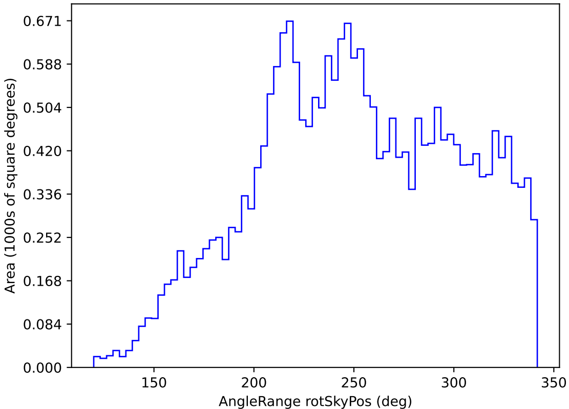
weather_cloudso14v3.4_10yrs All sky y band: AngleRange rotSkyPos
