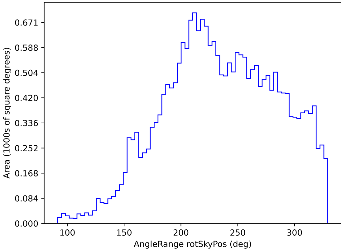
weather_cloudso14v3.4_10yrs All sky u band: AngleRange rotSkyPos
