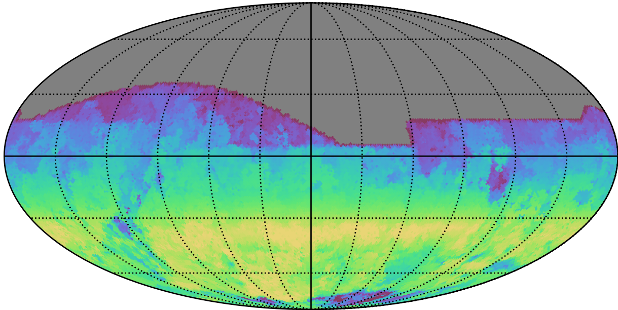
weather_cloudso14v3.4_10yrs All sky r band: AngleRange rotSkyPos
