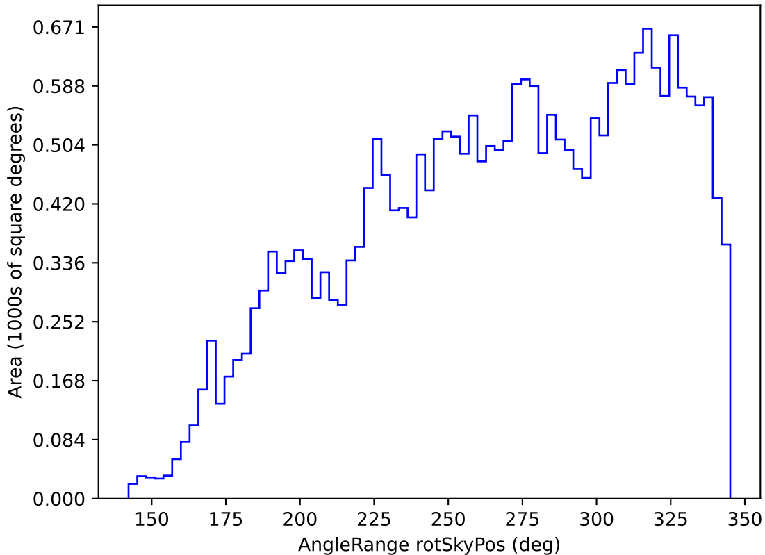
weather_cloudso14v3.4_10yrs All sky r band: AngleRange rotSkyPos
