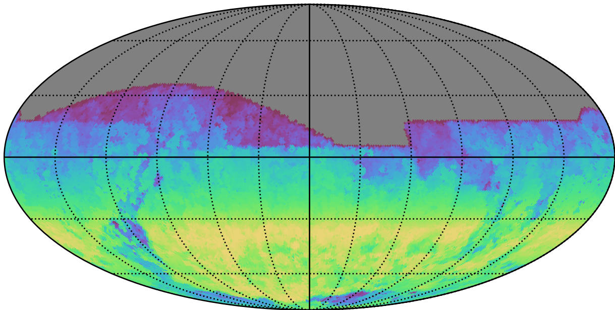
weather_cloudso14v3.4_10yrs All sky i band: AngleRange rotSkyPos
