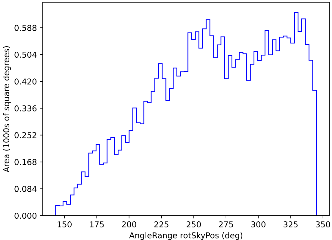
weather_cloudso14v3.4_10yrs All sky i band: AngleRange rotSkyPos
