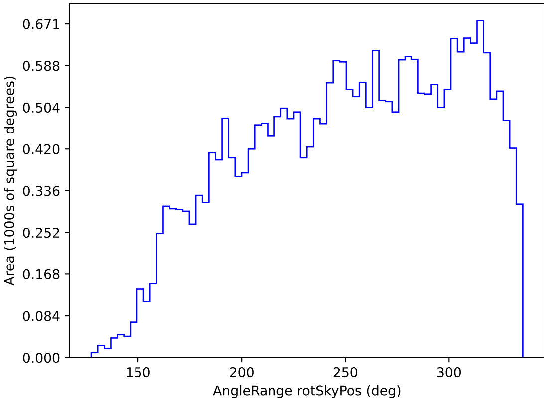
weather_cloudso14v3.4_10yrs All sky g band: AngleRange rotSkyPos
