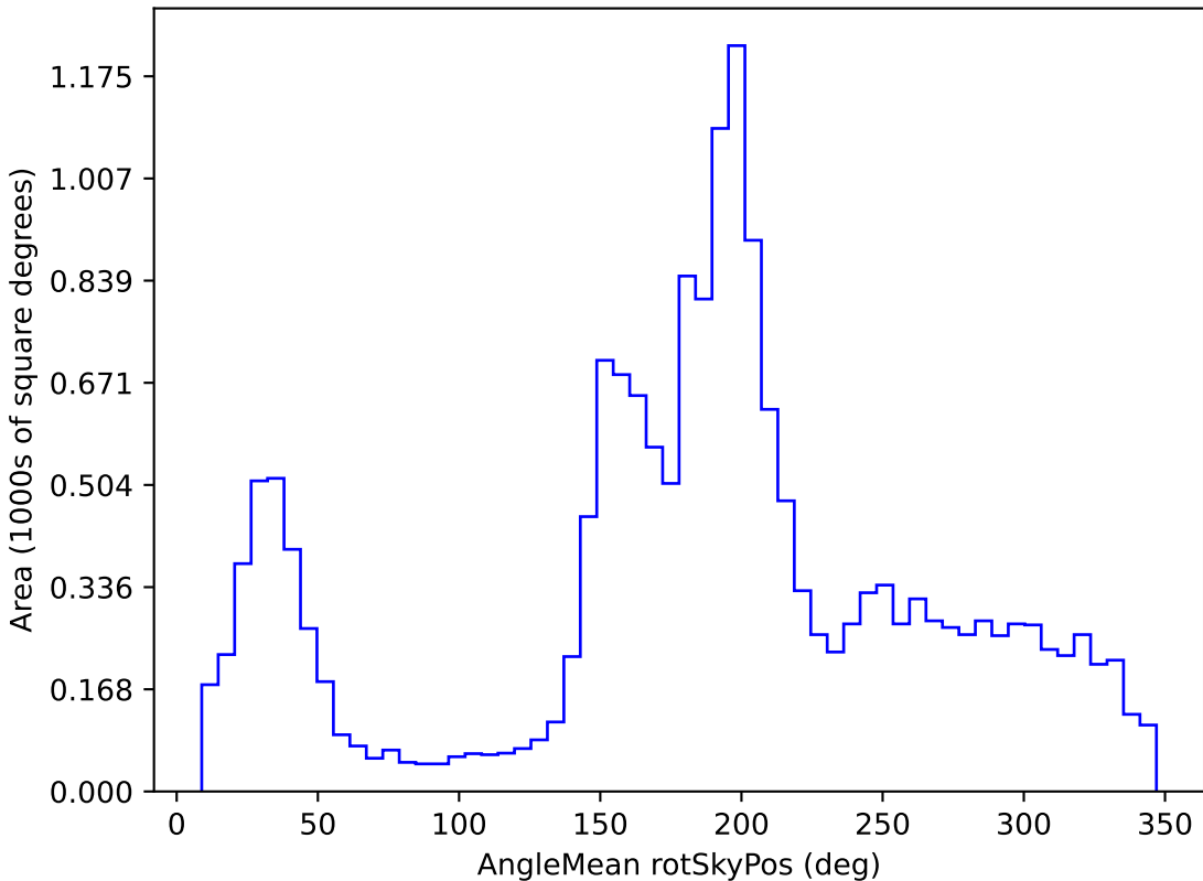
weather_cloudso14v3.4_10yrs WFD u band: AngleMean rotSkyPos
