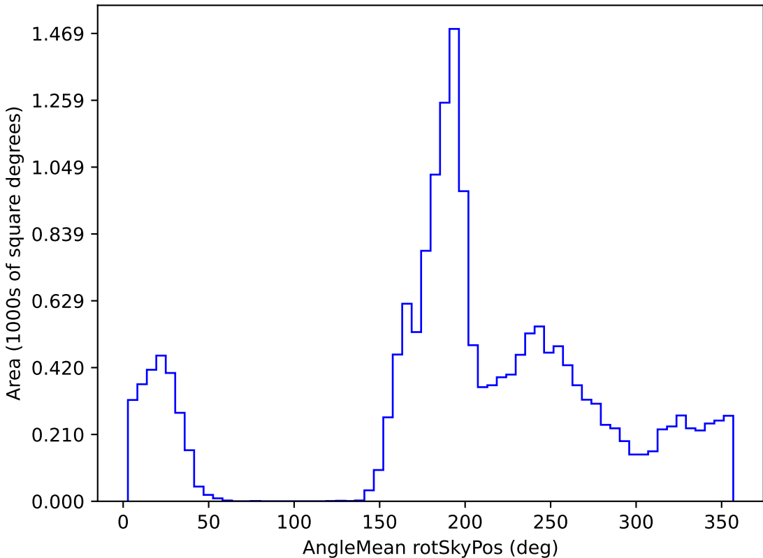
weather_cloudso14v3.4_10yrs WFD i band: AngleMean rotSkyPos
