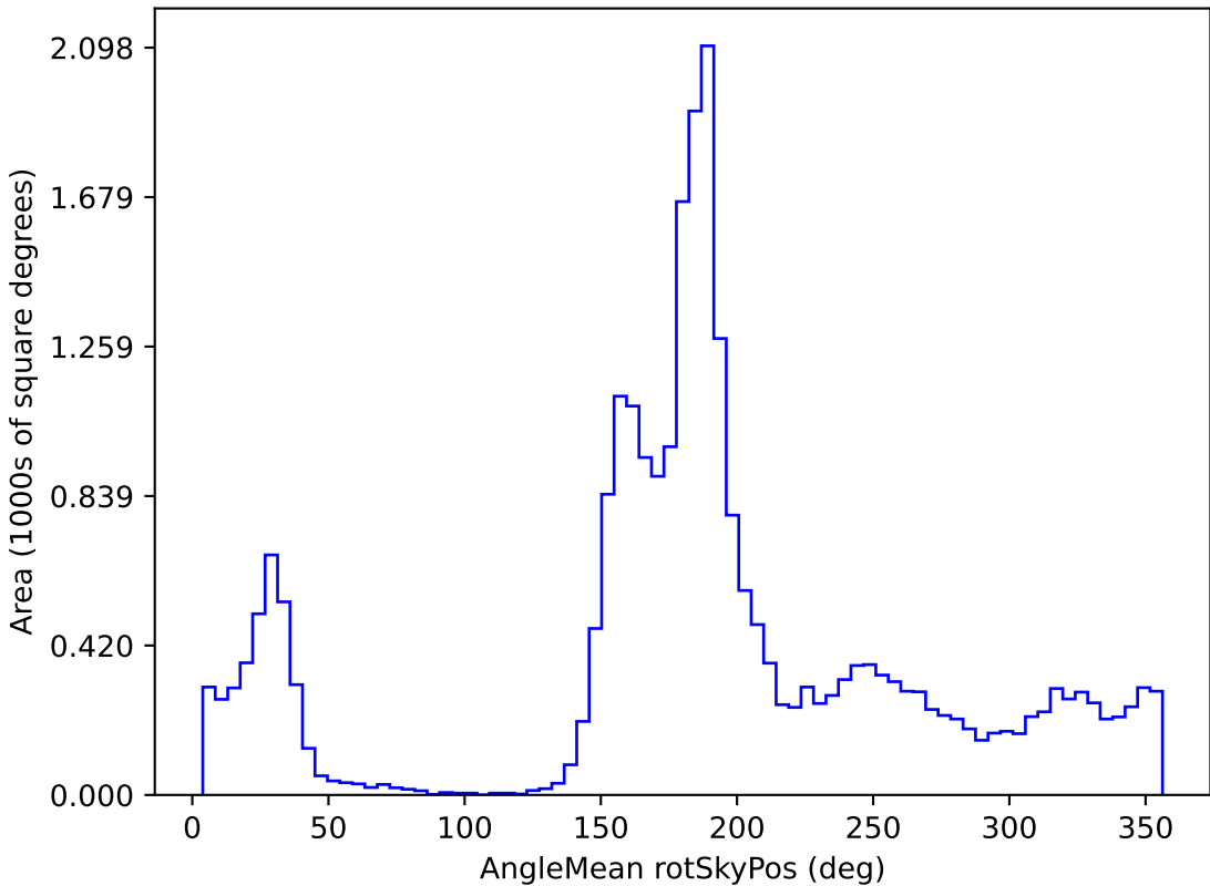
weather_cloudso14v3.4_10yrs All sky r band: AngleMean rotSkyPos
