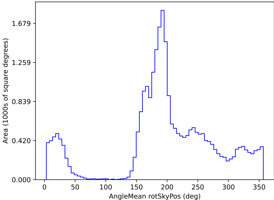
weather_cloudso14v3.4_10yrs All sky i band: AngleMean rotSkyPos
