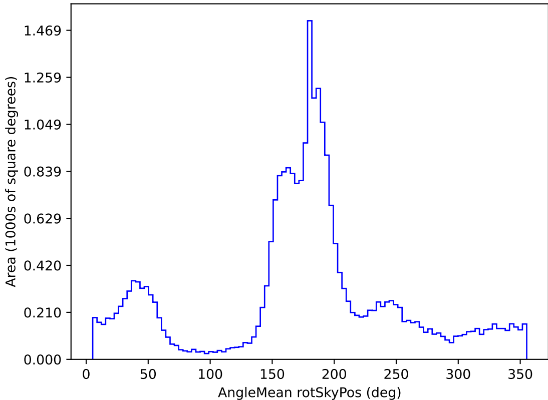
weather_cloudso14v3.4_10yrs All sky g band: AngleMean rotSkyPos
