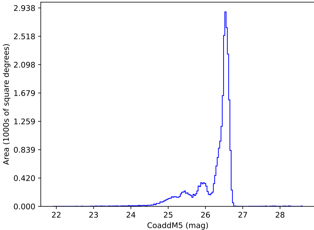
weather_cloudso14v3.4_10yrs i: CoaddM5
