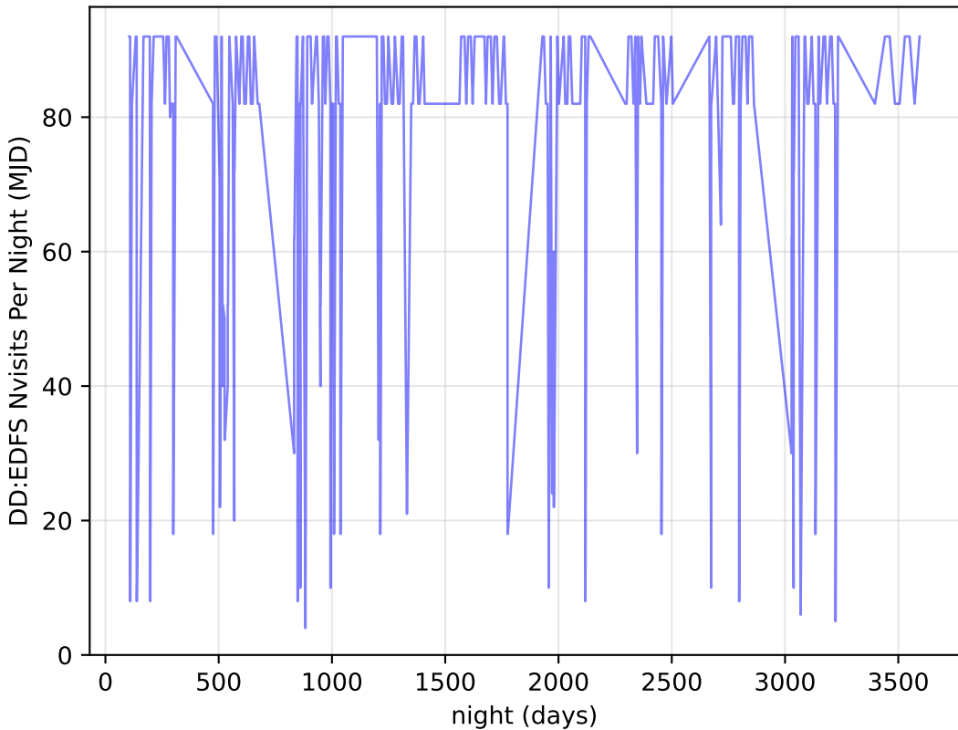
weather_cloudso14v3.4_10yrs all bands: DD:EDFS Nvisits Per Night
