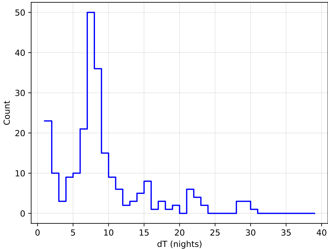
weather_cloudso14v3.4_10yrs all bands: DD:EDFS Delta Nights Histogram
