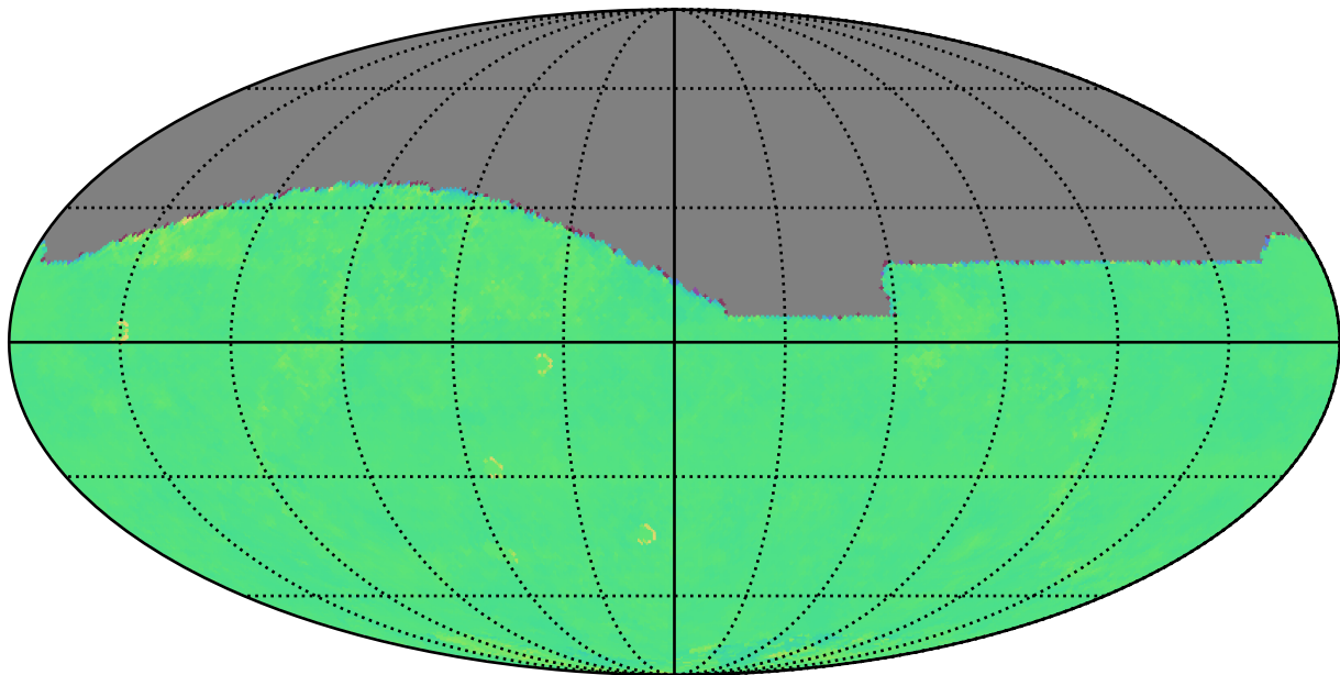
weather_cloudso12v3.5_10yrs z: Kuiper rotTelPos
