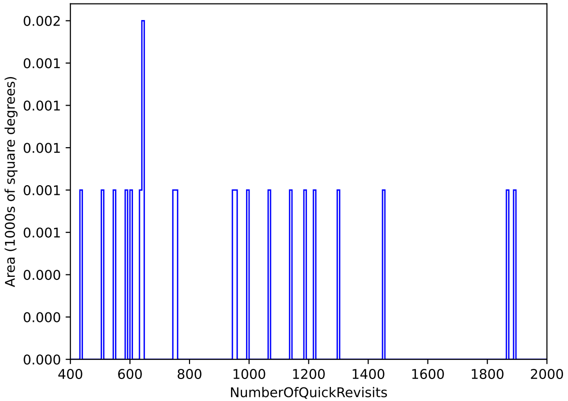
weather_cloudso12v3.4_10yrs : NumberOfQuickRevisits
