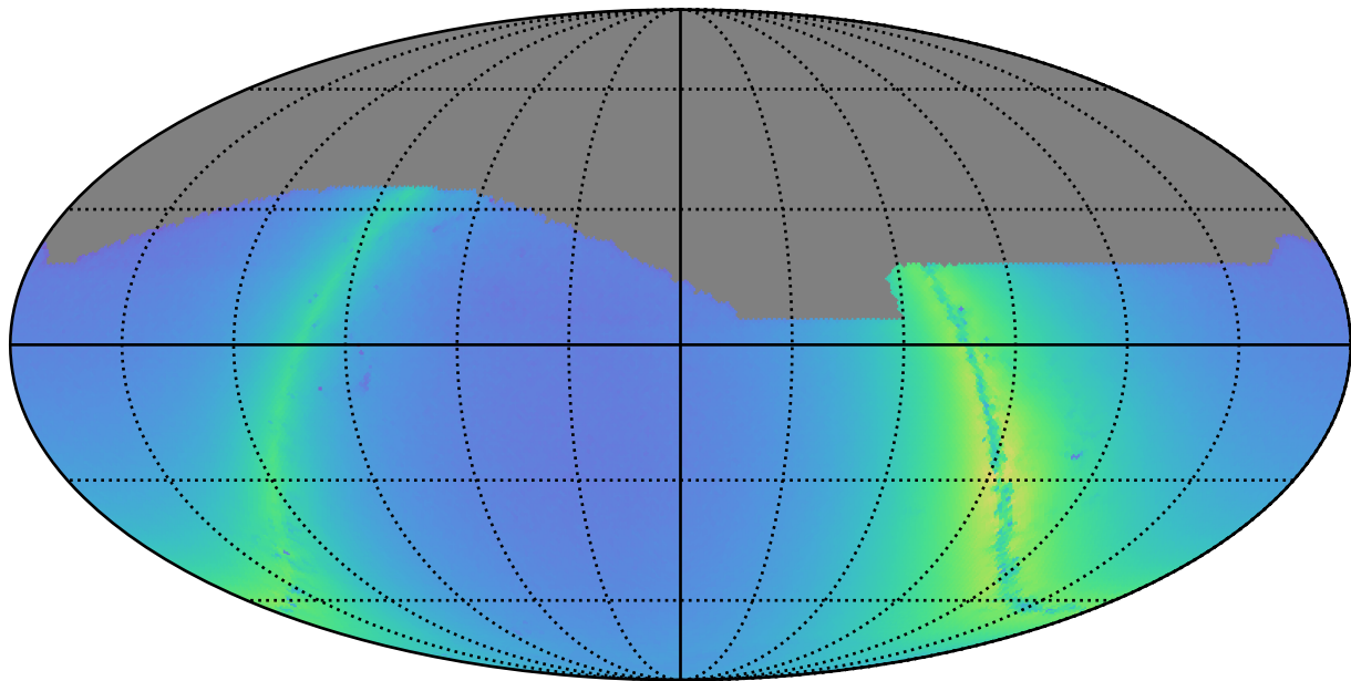
weather_cloudso12v3.4_10yrs i: Nstars_no_crowding
