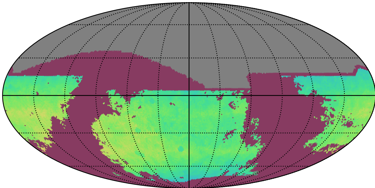
weather_cloudso12v3.4_10yrs i: NgalScale
