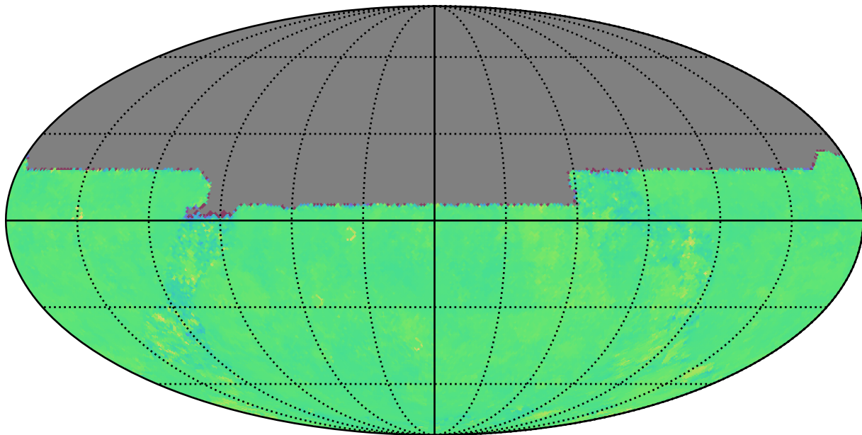
weather_cloudso12v3.4_10yrs u: Kuiper rotTelPos
