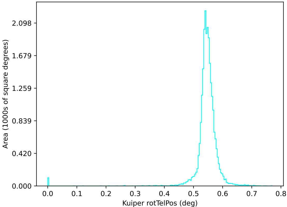
weather_cloudso12v3.4_10yrs u: Kuiper rotTelPos
