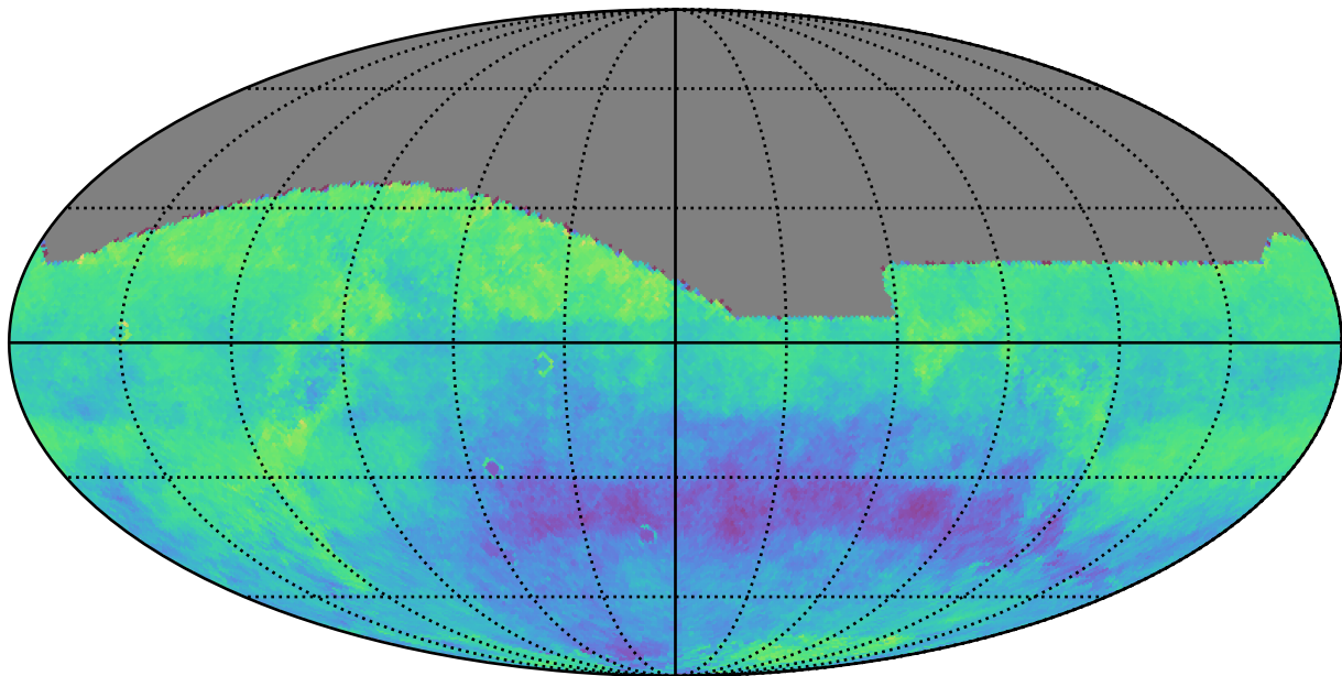
weather_cloudso12v3.4_10yrs z: Kuiper rotSkyPos
