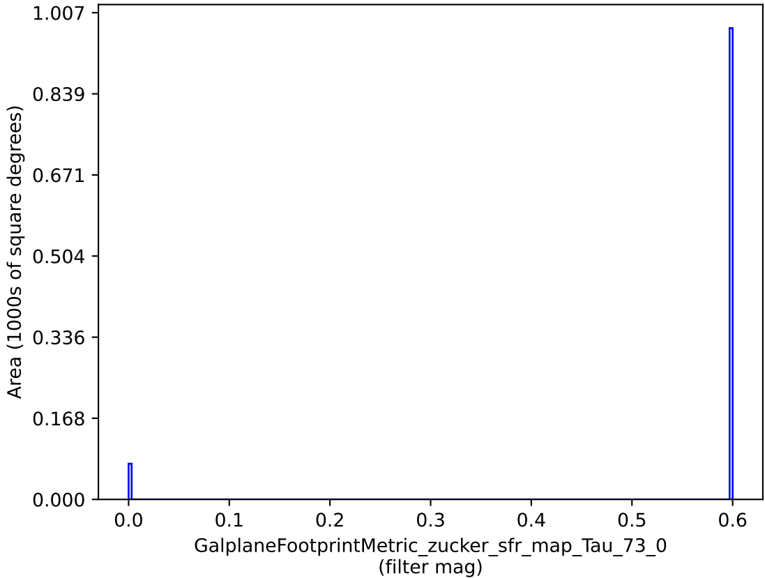
weather_cloudso12v3.4_10yrs : GalplaneFootprintMetric_zucker_sfr_map_Tau_73_0
