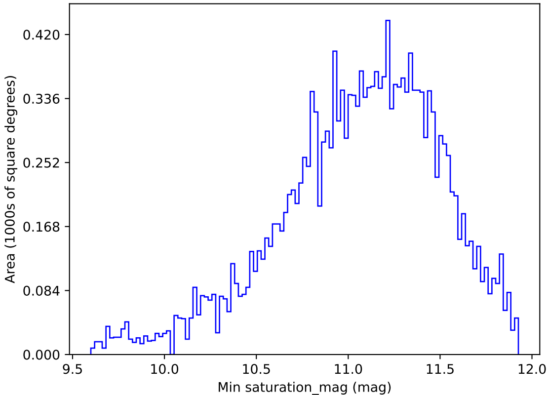
weather_cloudso12v3.4_10yrs WFD y band: Min saturation_mag
