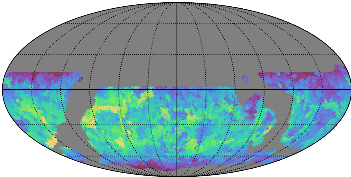
weather_cloudso12v3.4_10yrs WFD y band: Max saturation_mag
