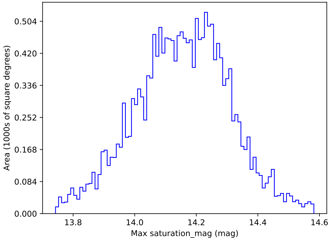
weather_cloudso12v3.4_10yrs WFD y band: Max saturation_mag
