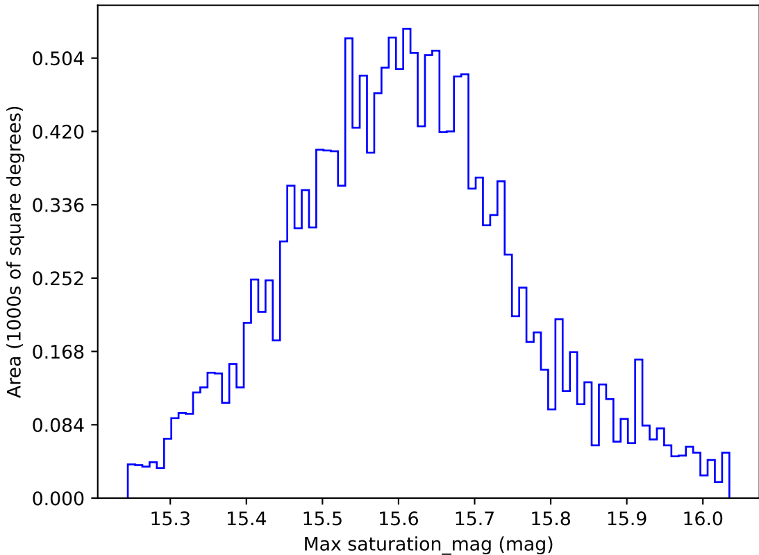
weather_cloudso12v3.4_10yrs WFD i band: Max saturation_mag
