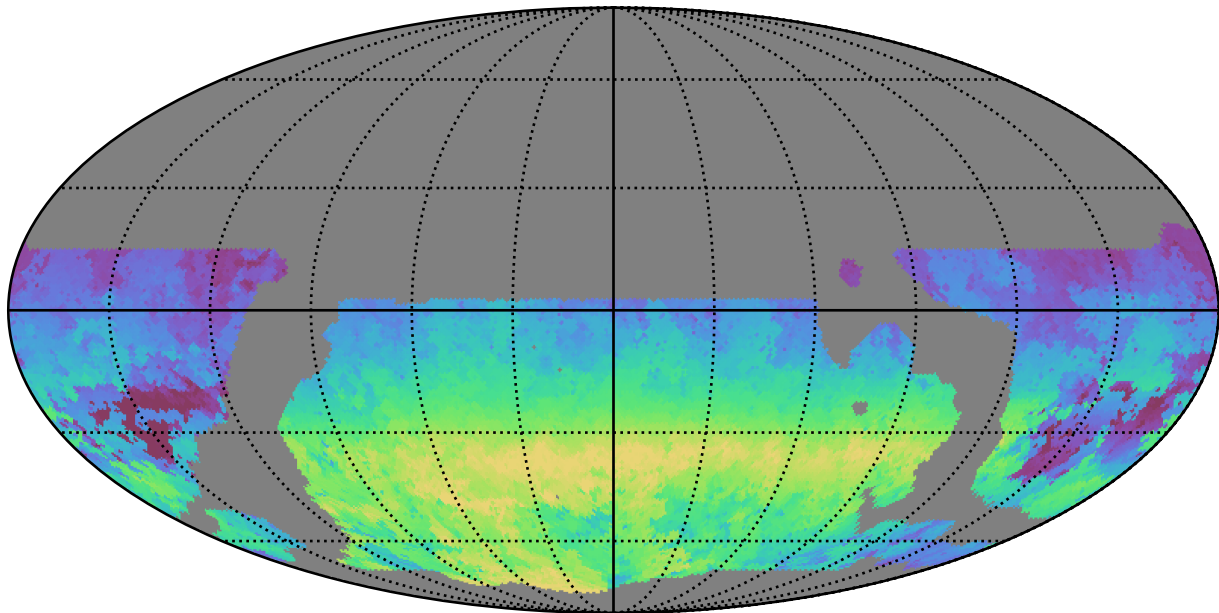
weather_cloudso12v3.4_10yrs WFD y band: AngleRange rotSkyPos
